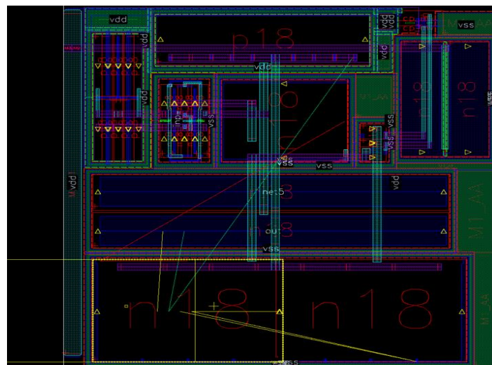
连接飞线
